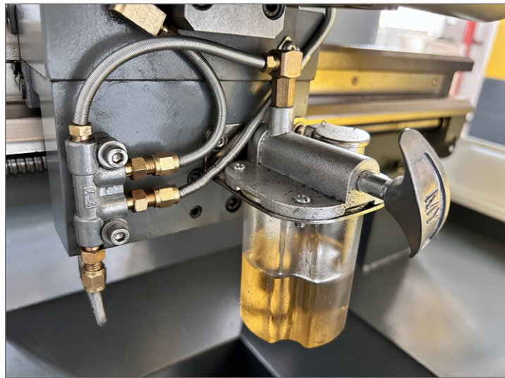
润滑系统
